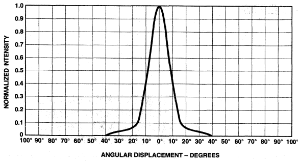
Figure 8. HLMP-Q106/-Q156.
