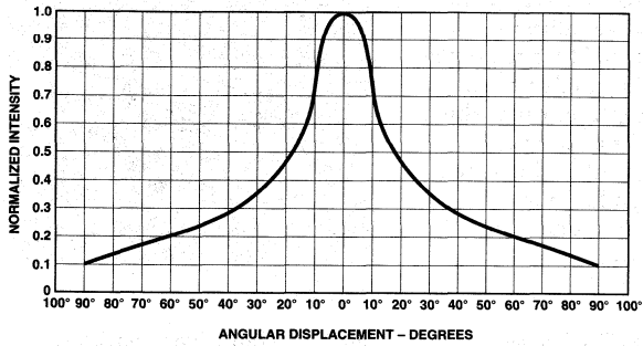
Figure 9. HLMP-Q102/-Q152
